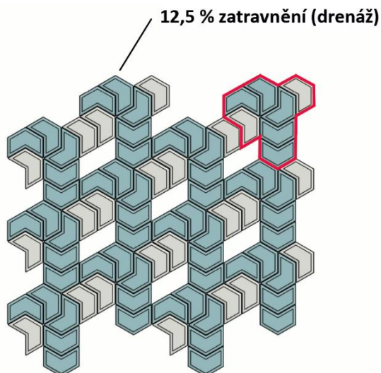
Skladba DITON OMNIA 19
