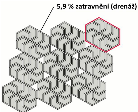
Skladba DITON OMNIA 11
