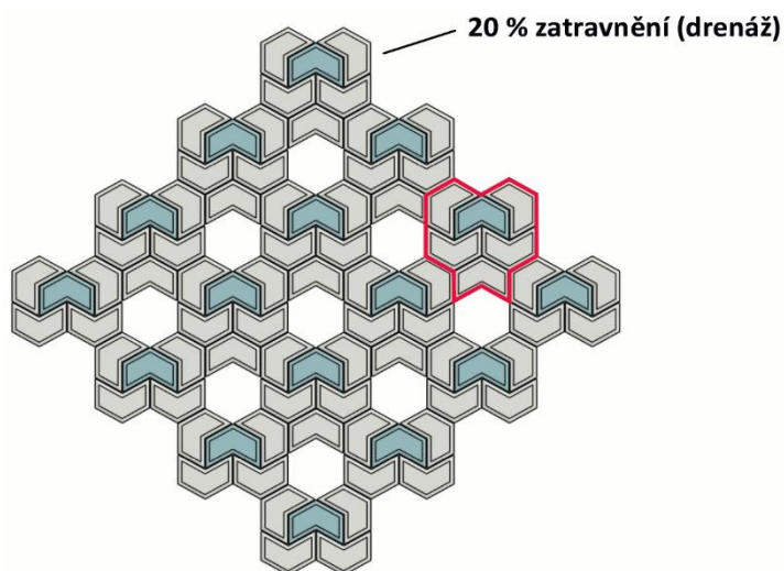
Skladba DITON OMNIA 30
