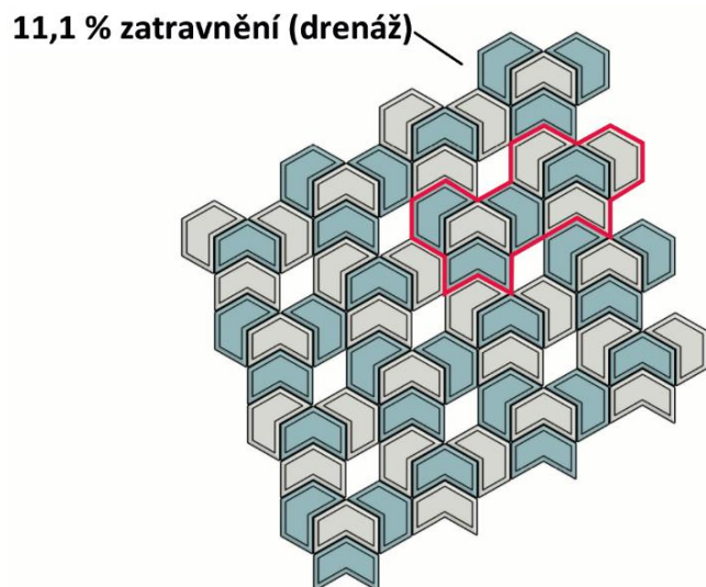
Skladba DITON OMNIA 13
