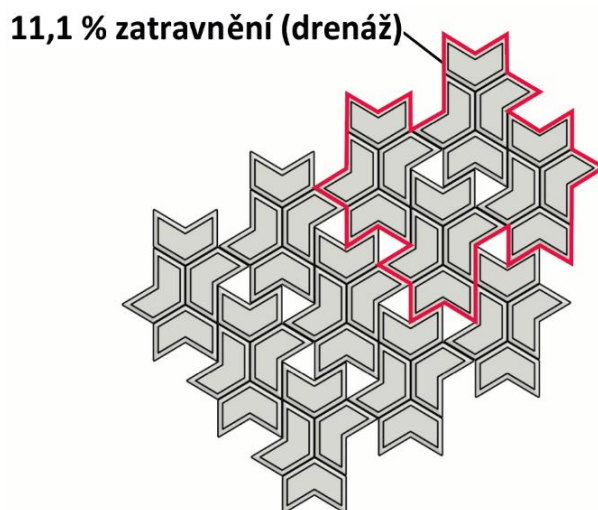
Skladba DITON OMNIA 14
