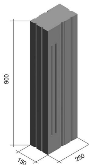
Obr. č. 11 – Palisáda D90 / 25 Dub
