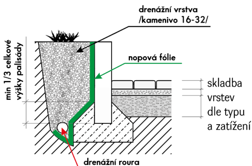
Obr. č.7 Uložení palisád do betonového lože
