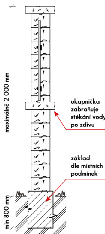
Obr. č. 6 Příklad plotové konstrukce
