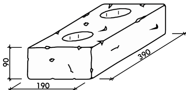
Obr. č. 7 Zdicí blok History – nízký kámen s otvory
