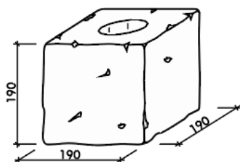
Obr. č. 9 Zdicí blok History - základní kámen poloviční
