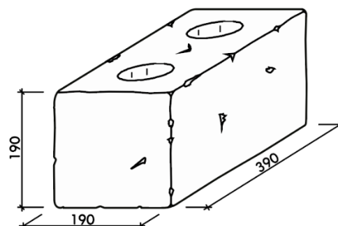
Obr. č. 10 Zdicí blok History základní kámen
