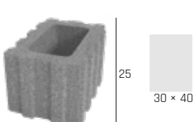
SVAHOVÁ TVÁRNICA QUADRA MALÁ Rozmery: 30 × 40 × 25 cm
