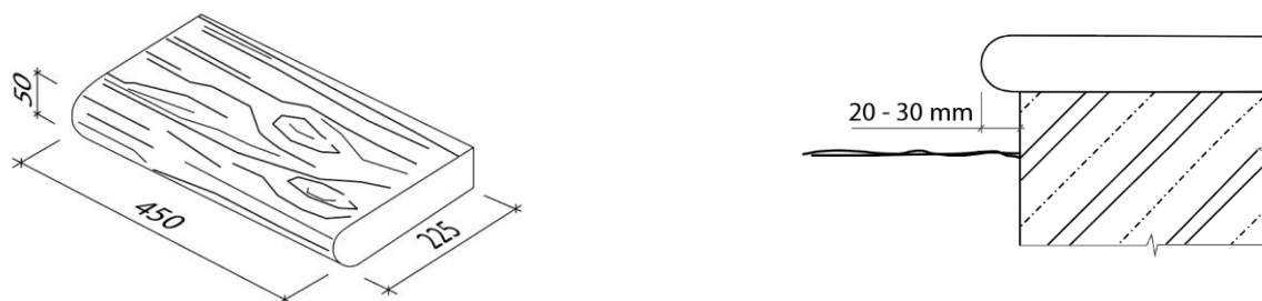
Obr. č. 9 – Detail přesahu bazénových lemů
