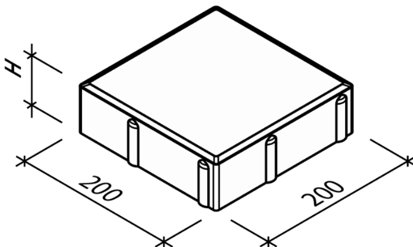
Obr. č. 11 – Kostka AQUAPORE rozměry
