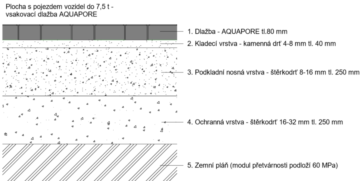
Obr. č. 15 – Příklad skladby podloží pro dlažbu do 7,5 t
