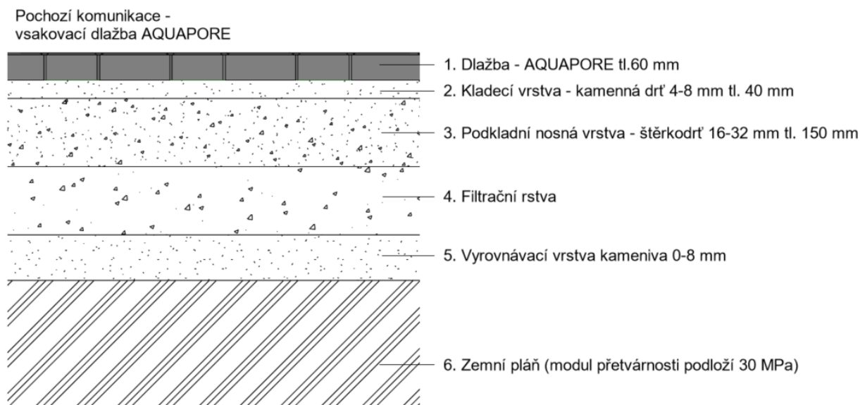
Obr. č. 12 – Příklad skladby podloží pro dlažbu pochozí
