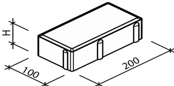
Obr. č. 9 – Parketa AQUAPORE rozměry
