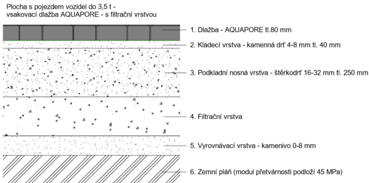
Obr. č. 14 – Příklad skladby podloží pro dlažbu do 3,5 t s filtrační vrstvou
