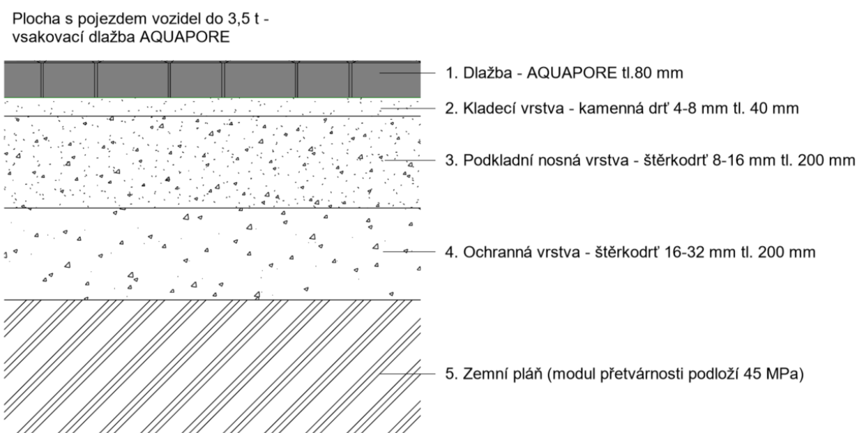
Obr. č. 13 – Příklad skladby podloží pro dlažbu do 3,5 t
