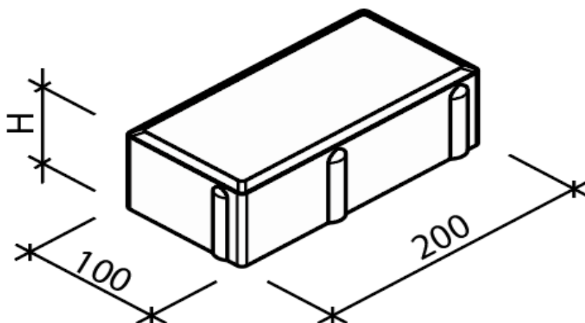
Obr. č. 8 – Parketa AQUAPORE rozměry
