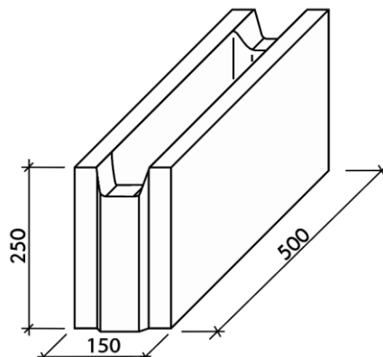
Obr. č. 10 Ztracené bednění 15
