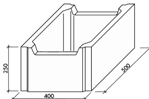
Obr. č. 14 Ztracené bednění 40
