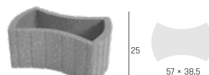
SVÁHOVÁ TVÁRNICE OKTÁVA Rozměry: 57 × 38,5 × 25 cm
