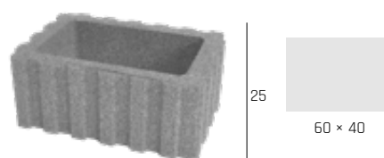
SVÁHOVÁ TVÁRNICE QUADRA VELKÁ Rozměry: 60 × 40 × 25 cm
