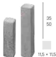
PALISÁDA POLO 35 Rozměry: 11,5 × 11,5 × 35 cm
