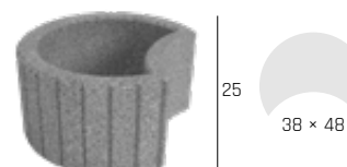
SVÁHOVÁ TVÁRNICE DELTA VELKÁ Rozměry: 38 × 48 × 25 cm
