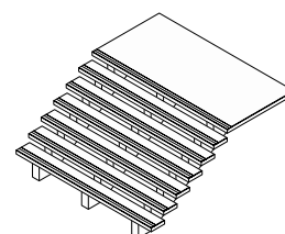
SCHODISKOVÝ SYSTÉM ŠÍRKY 2,50 - 3,00 M
