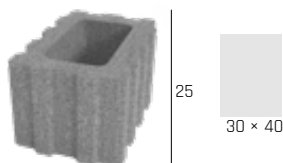
SVAHOVÁ TVÁRNICA QUADRA MALÁ Rozmery: 30 × 40 × 25 cm
