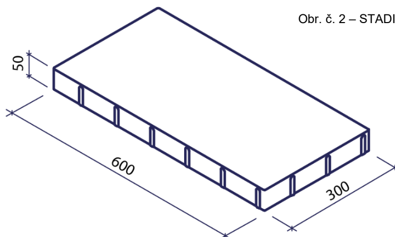
Stadio 60 / 30 / 5 – Skladebné rozměry
