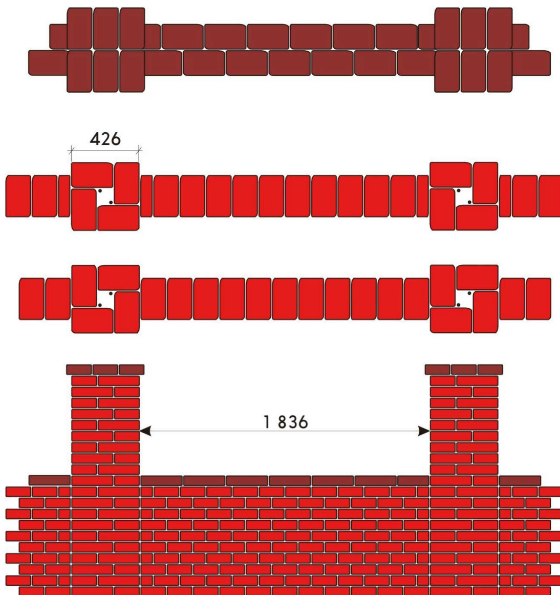
Obr. č.3 – Návrh plotu ze zdicích prvků Cihla hladká II. (Cihla History II.) o šířce 260 mm
