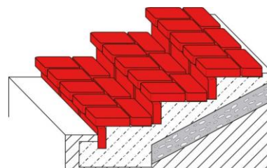
Šířka schodiště 800 mm
