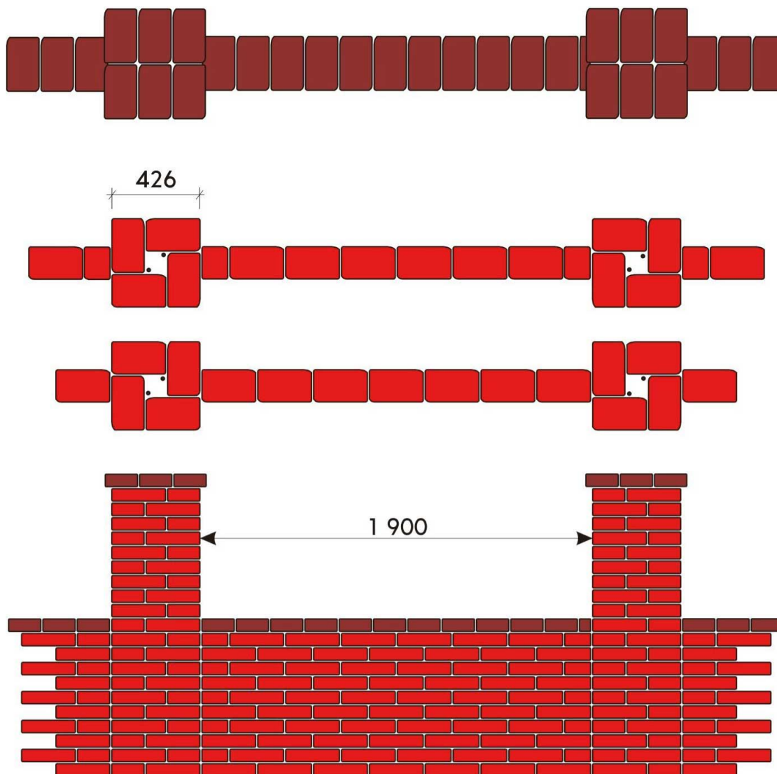
Obr. č.1 – Návrh plotu ze zdicích prvků Cihla hladká II. (Cihla History II.) o šířce 156 mm
