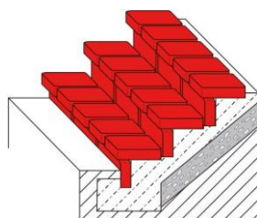
Šířka schodiště 800 mm
