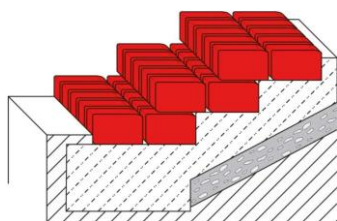
Šířka schodiště 340 mm
