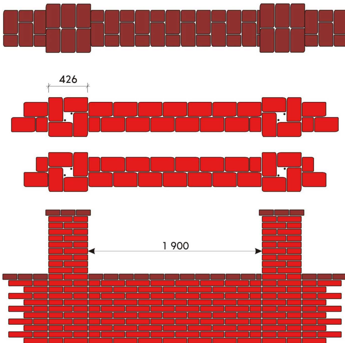
Obr. č.2 – Návrh plotu ze zdicích prvků Cihla hladká II. (Cihla History II.) o šířce 322 mm
