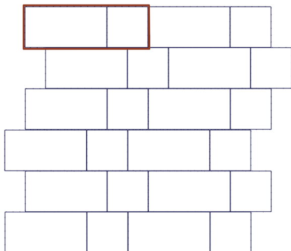
Skladba Monaco 5
