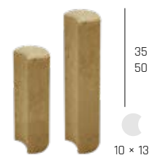
PALISÁDA GRANDE 120 Rozmery: 17,5 × 20 × 120 cm
