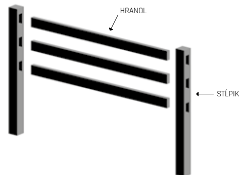
FARMÁRSKY PLOT - STĽPIK A Rozmery: 13 × 13 × 70 cm
